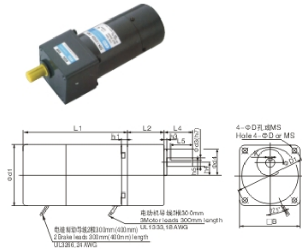
6~40W无励磁动作型电磁制动电动机整机外形图
