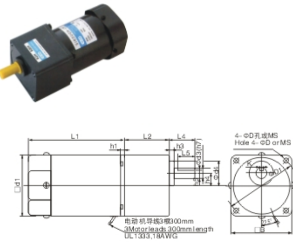
60~180W感应减速电动机整机外形图 60~180W Induction gear motor dimension
