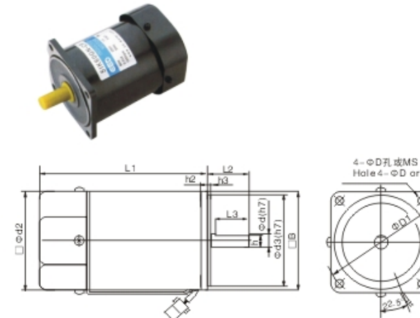
60~180W调速电动机光机外形图
