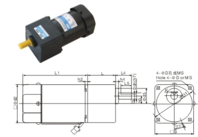
60~180W调速电动机整机外形图
