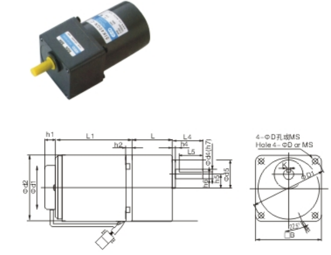
6~40W调速电动机整机外形图
