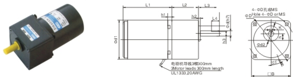
转矩减速电动机整机外形图 Torque gear motor dimension
