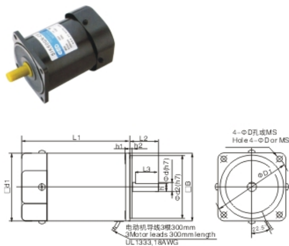
60~180W感应电动机光机外形图 60~180W Induction bare motor dimension
