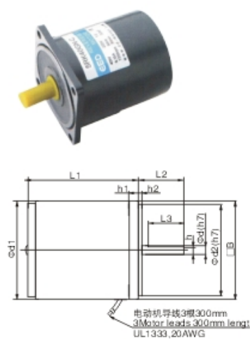
6~40W可逆电动机光机外形图
