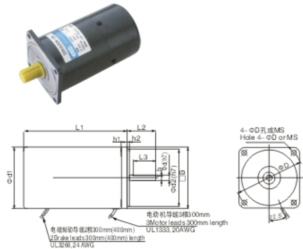
60~180W无励磁动作型电磁制动电动机光机外形图
