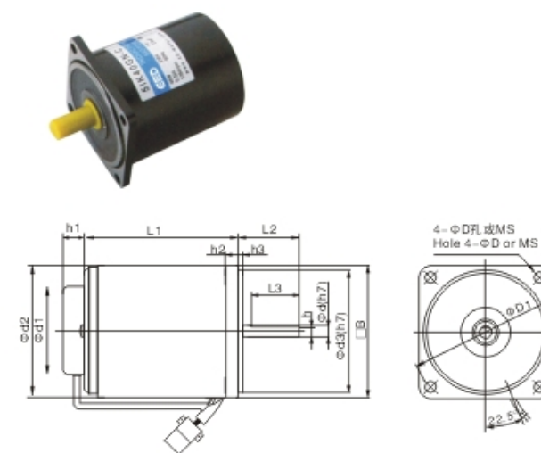
6~40W调速电动机光机外形图
